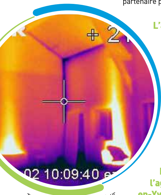
Thermographie réalisée à l'intérieur d'un bâtiment par l'ALEC SQY
